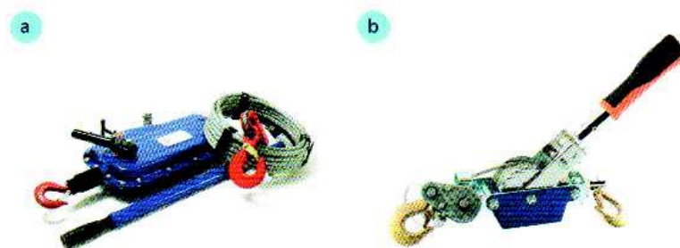
Ryc. 31.3. Rodzaje ciągników: (a) wciągarka, (b) przyciągarka
