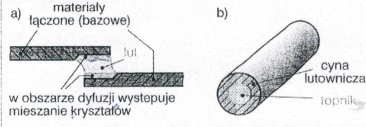
Rys. 1. a) Połączenie lutowane, b) Drut lutowniczy (tino)
