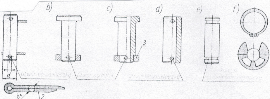
rys. 4.38. Sworznie: a) gładki pełny, b) kształtowy pełny, c) kształtowy drażony, d) gładki ażony, e) rowkowy, f) pierścienie osadzone sprężynujące — podkładka, 2 — zawłczka, 3 — pierścień
