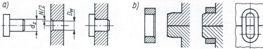
Rys. 4.1. Połączenia wciskowe: a) bezpośrednie, b) pośrednie
