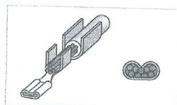
Rys. 3. Połączenie krepowane (jednostronne formowanie materiału przez zagięcie tapek tulejki)
