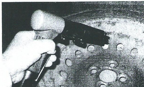
Rys. 1. Pistolet iglicowy
