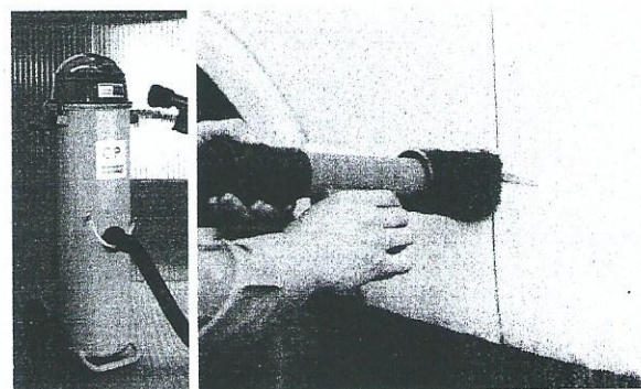
Rys. 2. Urządzenie do piaskowania
