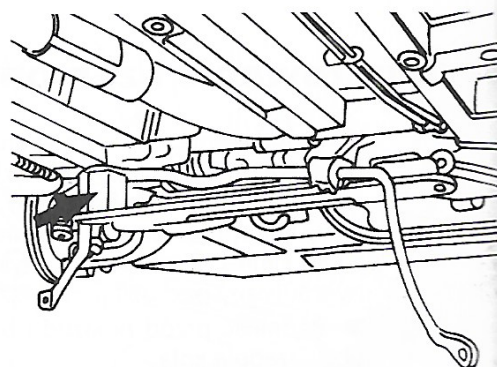
Rys. 7.18. MONTOWANIE DRAŻKA STABILIZATORA DO NADWOZIA. Klocek drewniany, wskazany strzałką, podłożony pod drążek stabilizatora, ułatwia jego ufatwianie montaż
