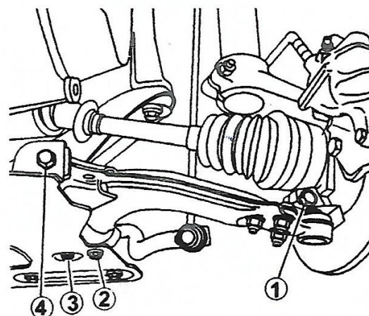
Rys. 7.14. MOCOWANIE WAHACZA POPRZECZNEGO (opis w tekście)
